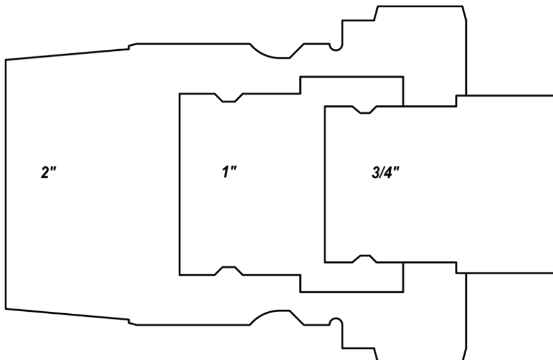
Dixon ST-Series
