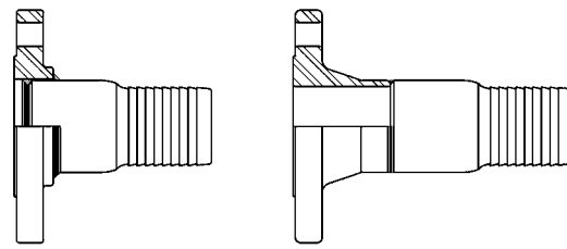
Свободный фланец с выступом
