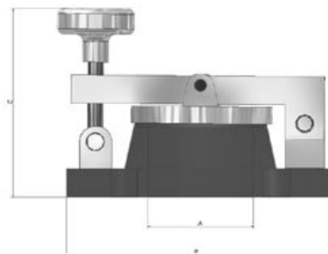
Размеры для опускания с помощью винта
