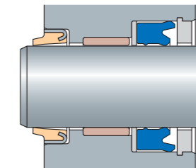
Монтаж в открытой канавке
