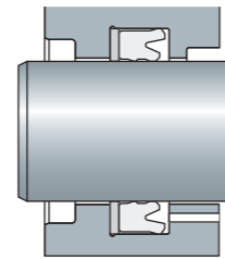
Пример монтажа STR-D/A
