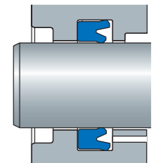
Пример монтажа
