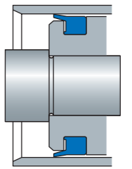
Пример монтажа
