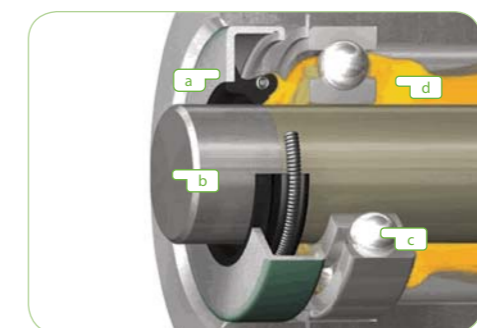
a: Манжетное уплотнение b: Вал c: Подшипник d: Смазка
