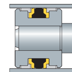
Пример монтажа
