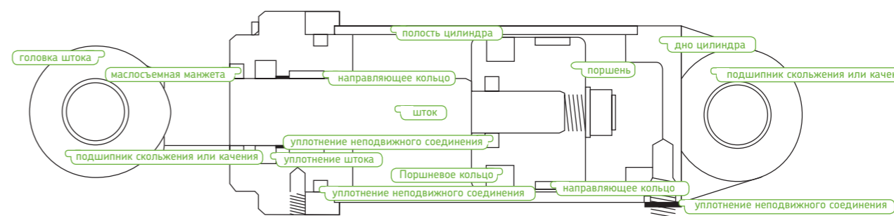
Гидравлический цилиндр – Терминология
