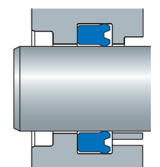
Пример монтажа
