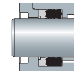
Пример монтажа
