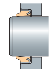
Пример монтажа PA
