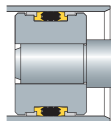
Пример монтажа
